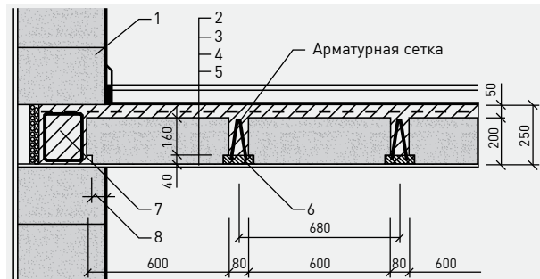
Сечение конструкции перекрытия перпендикулярно оси балки
