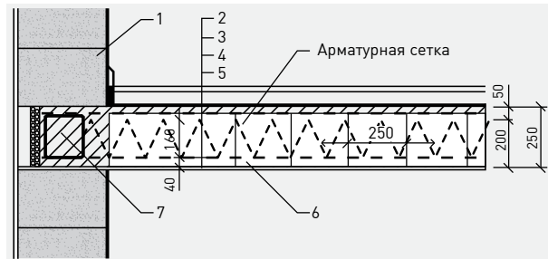
Сечение конструкции перекрытия параллельно оси балки
